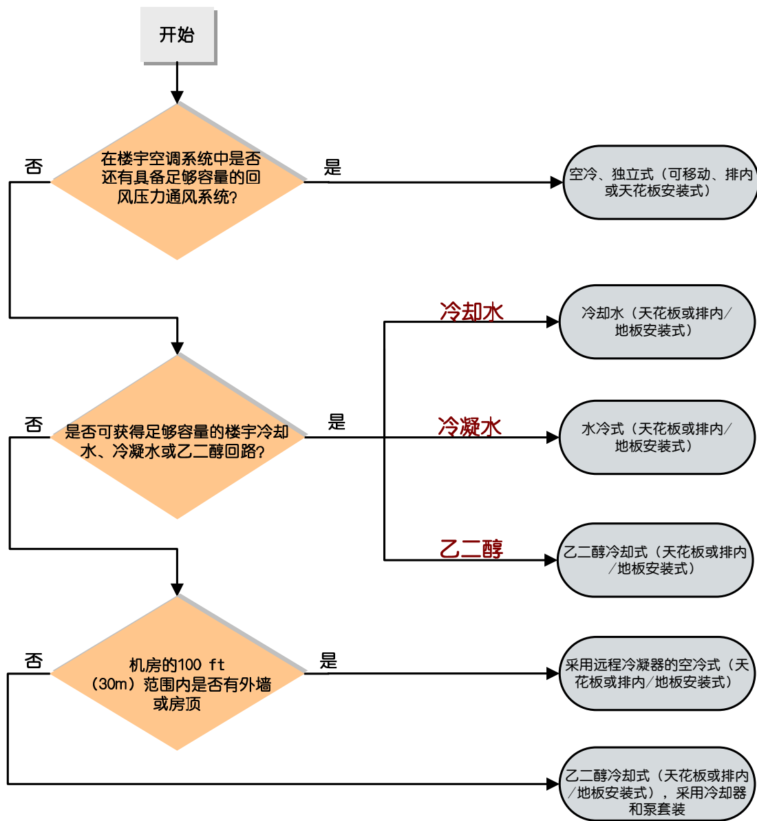
图 8 专用空调机选型
